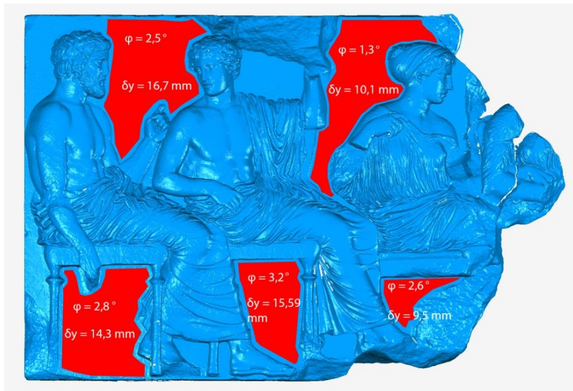
Τρισδιάστατο ψηφιακό μοντέλο του λίθου VI της ανατολικής ζωφόρου με ενδείξεις των αποκλίσεων από την κατακόρυφο του εδάφους του αναγλύφου.
